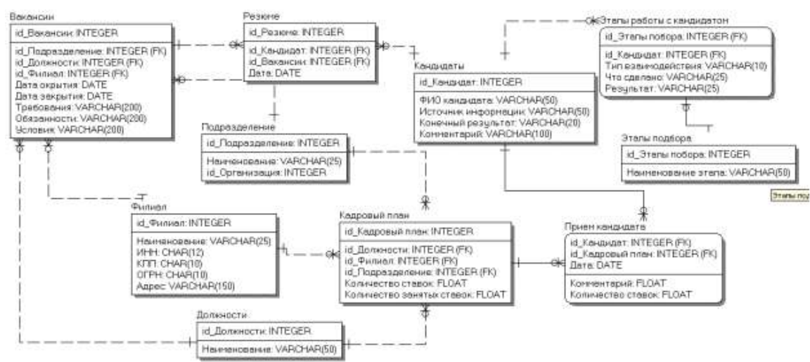
Рисунок 12 – Физическая модель данных
