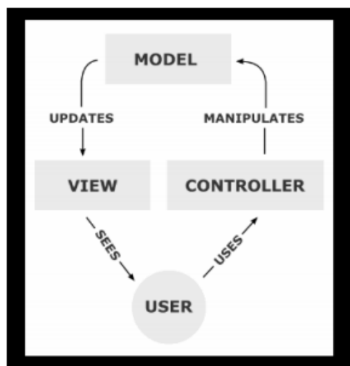
Рисунок 13 – Модель MVC
