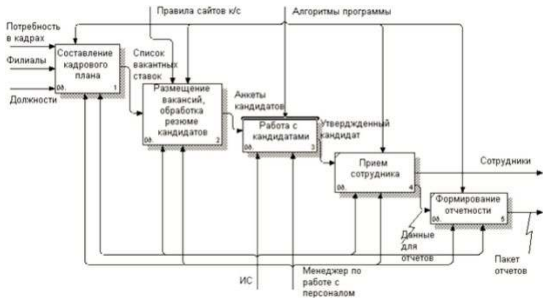
Рисунок 6 – Декомпозиция контекстной диаграммы
