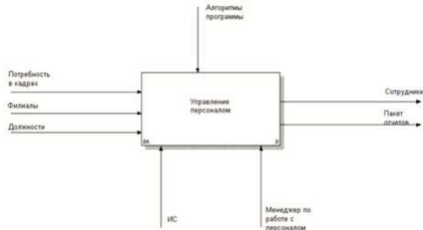
Рисунок 5 – Контекстная диаграмма информационной системы
