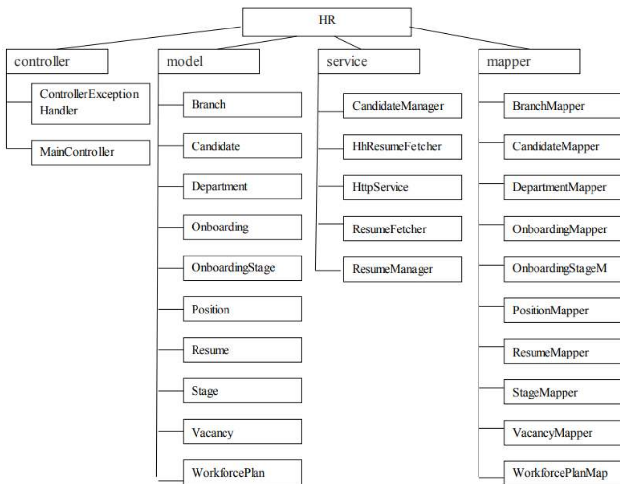
Рисунок 14 – Структурная схема пакетов документов
