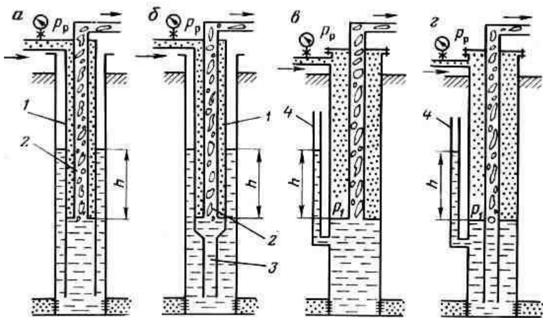
Рис. 9.2. Схема конструкций газлифтных подъемников: а - двухрядный подъемник, б - полутораярный подъемник, в - однорядный подъемник, г - однорядный подъемник с рабочим отверстием
